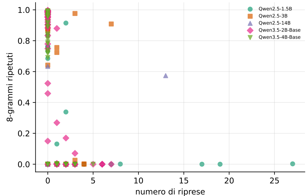
8-grammi ripetuti vs riprese \rho=-0.66 , p=0.000 — correlato: da approfondire
