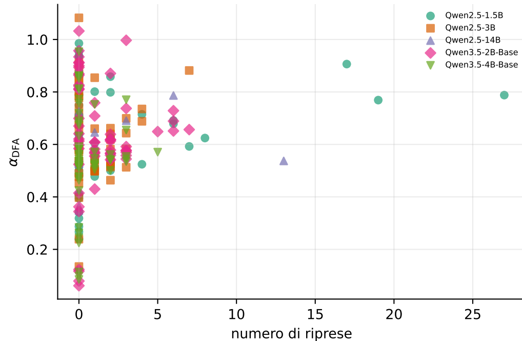
\alpha_{DFA} vs riprese \rho=+0.03 , p=0.632 — nessun artefatto
